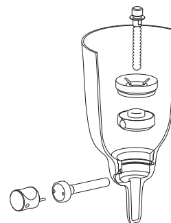
Icelock Ratchet 621
